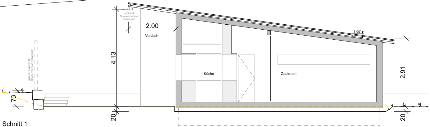
Schnitt 1
