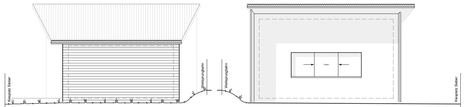
Ansicht Kiesplatz
