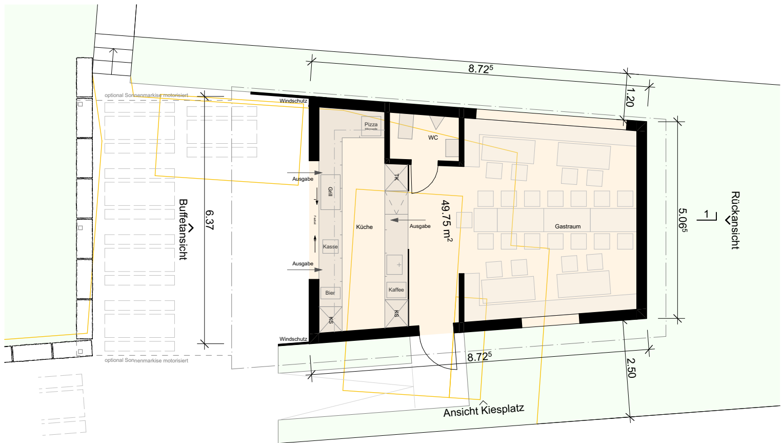
Grundriss
